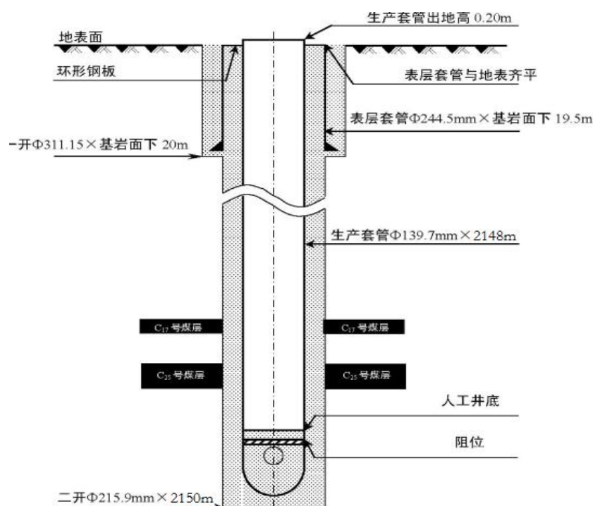
图 4 井身结构图
