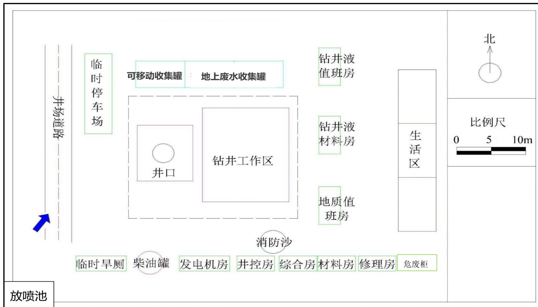
附图 3 项目井场平面布置图
